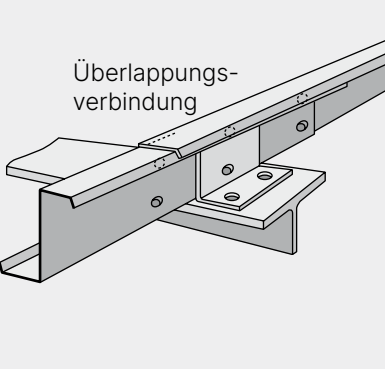
Z-Profil als Pfette
