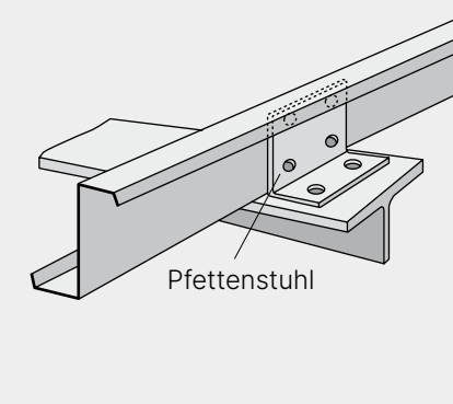
Z-Profil als Pfette
